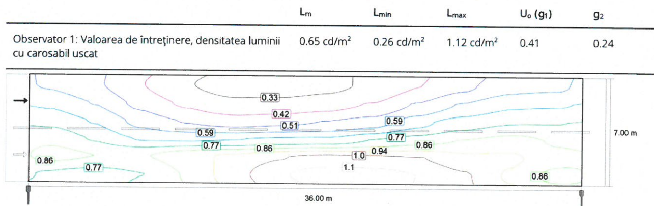
Observator 2: Valoarea de întreținere, densitatea luminii cu carosabil uscat [cd/m²] (Linii Isolux)
